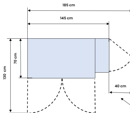
Vue de dessus de l'armoire SKALEX
