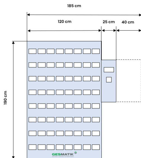
Vue de face de l'armoire SKALEX
